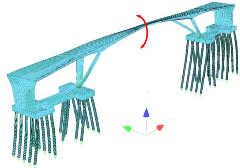
Figuur 104: f_2=1,58\text{Hz} – Torsie mode
