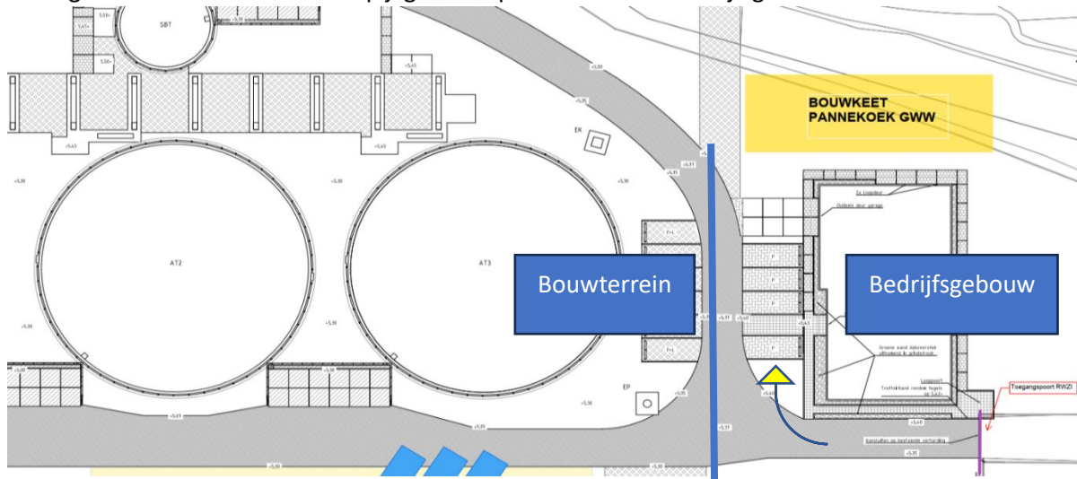
Plattegrond RWZI Terwolde. Gele pijl geeft looproute naar het bedrijfsgebouw aan.
